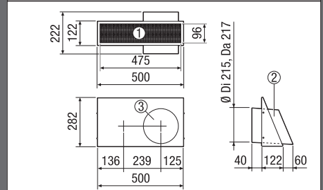
Technische Zeichnung
