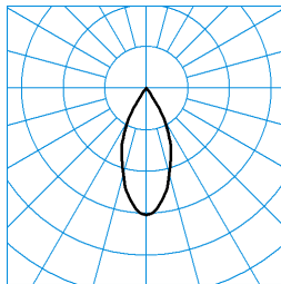
TX092394 UGR I = 18.1 UGR q = 18.1 DIN 5040: A80 UTE: 0,82 A ■ CO - C180
