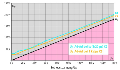
Schutzpegeldiagramm DBX U4 KT DB S 0-180
