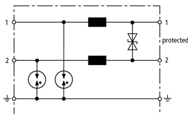
Principalschaltbild BVT ALD 36
