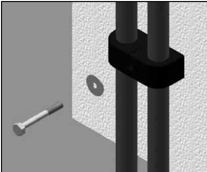
Abb. 5: Schellenkörper befestigen
