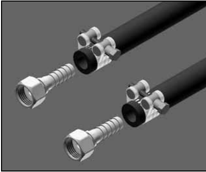
Abb. 4: Druckschläuche kürzen
