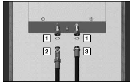
Abb. 3: Druckschläuche befestigen
