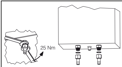
Abb. 1: Schlauchtülle entfernen
