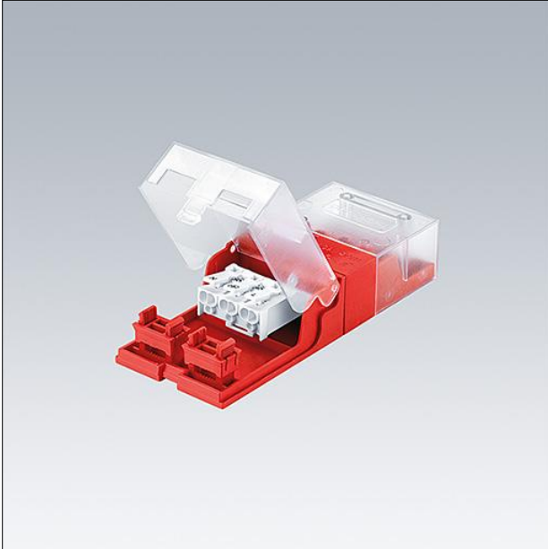
TE_CONNECTOR_F_3_pole_CLASS_I.jpg
