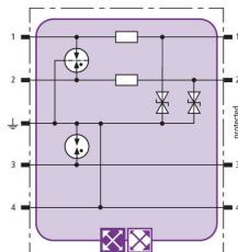
Prinzipschaltbild BXT ML2 BE S 24
