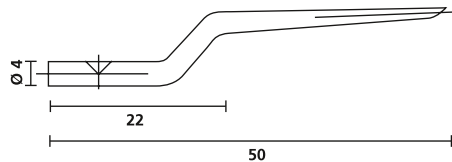
Ersatzdorne für NA1K/3
