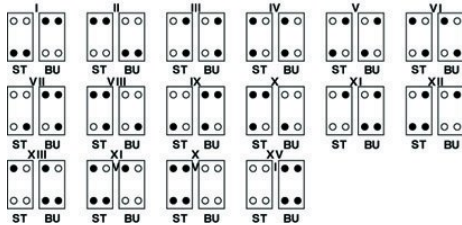
Codierung für Gehäuse mit einem Kontakteinsatz
