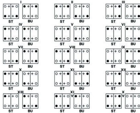
Codierung für Gehäuse mit zwei Kontakteinsätzen
