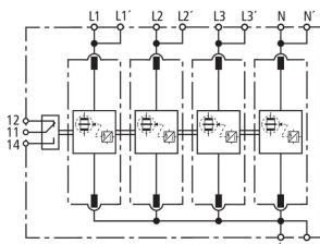
Prinzipialschaltbild DV M TNS 255 FM
